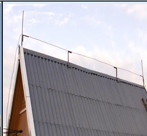
Тросовый молниеприемник.
